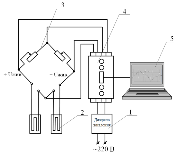
Рис. 2. Схема вимірювальної та реєструючої апаратури експериментальної установки
