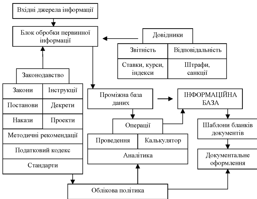
Рис. 1.15. Схематична структура облікової програми
