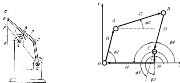
Рис.1. Структурна та кінематична схеми
