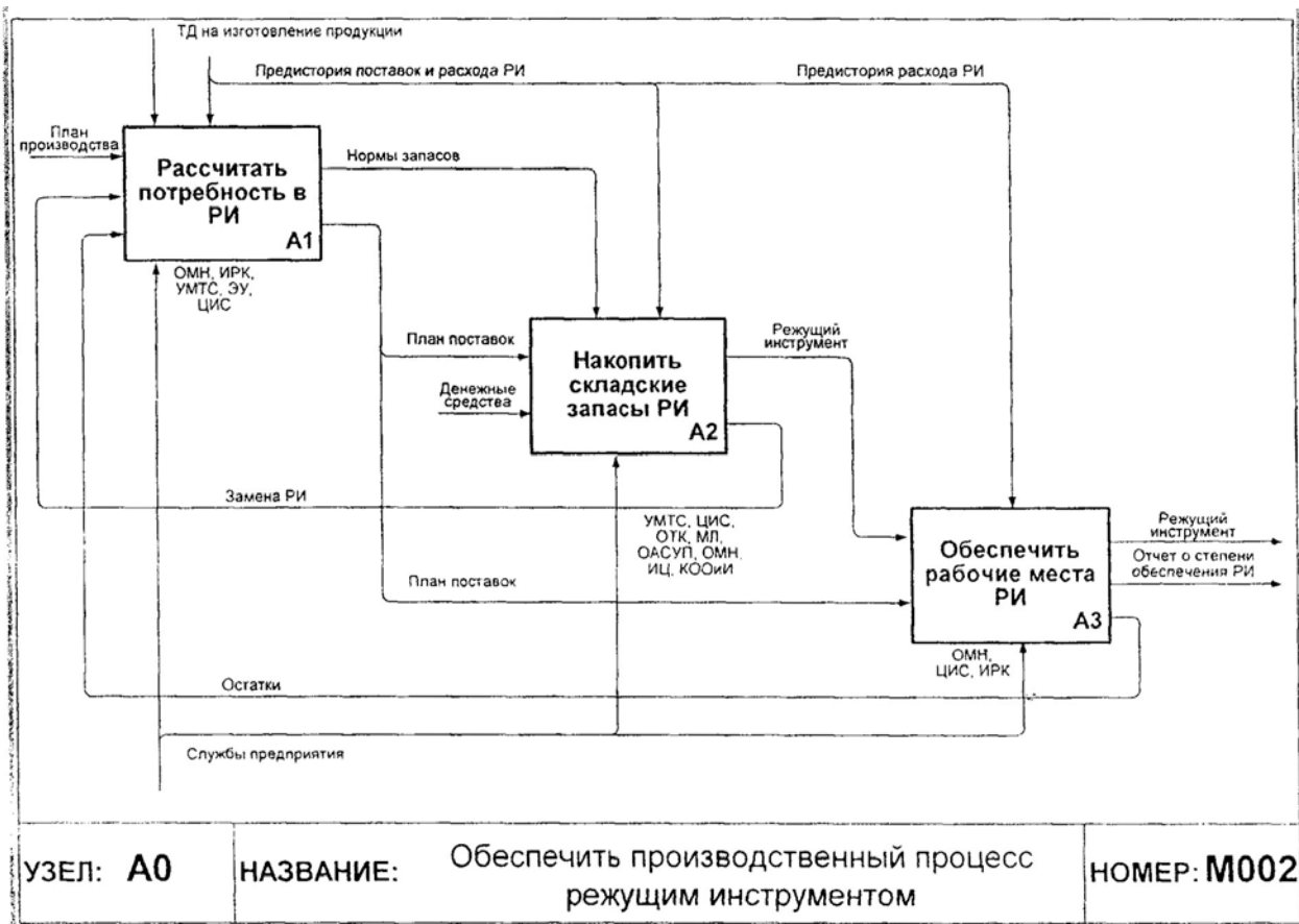
Рис. 2. SADT – DFD-модель функціональних взаємодій в процесі забезпечення виробництва різального інструменту
