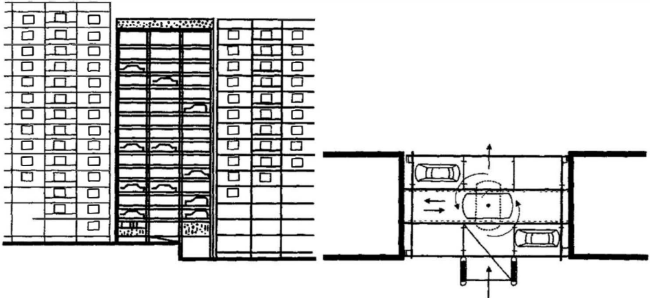
Рис. 3 Приклад прибудовування автоматизованої багатопверхової автостоянки до торцьової частини житлового будинку. Розріз, план
