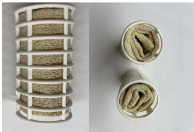
Рис. 5.2 - Касети з волокнистим матеріалом, наповненим мінеральним адсорбентом
