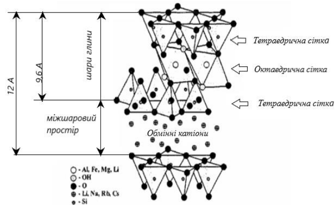
Рис. 2.5 – Структура монтморилоніту
