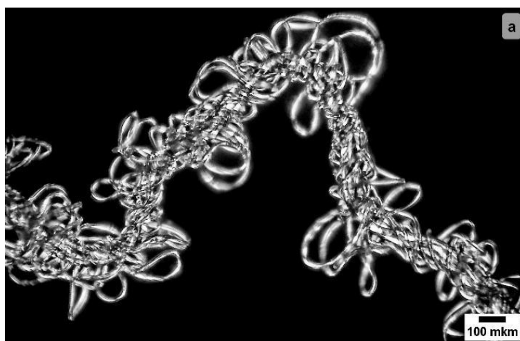
Рис. 3.1 – Мікрофотографія в поляризованому світлі вихідних комбінованих ПУ-ПА волокон
