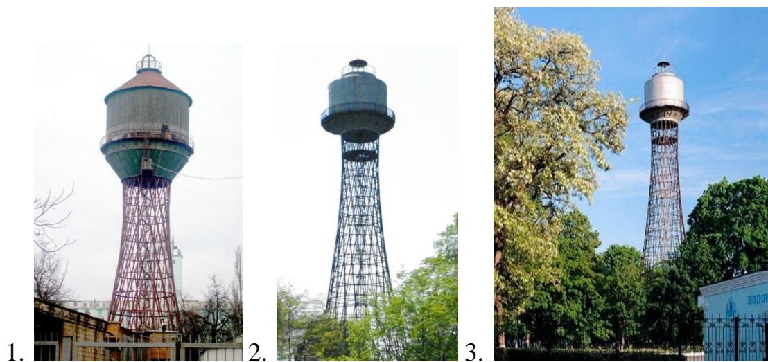
Рис. 6. Вежі В. Шухова в Україні: 1 - водонапірна вежа у м. Біла Церква (1929 р.); 2 - водонапірна вежа у м. Помошна (1934 р.); 3 - водонапірна вежа у м. Черкаси (1914 р.)
