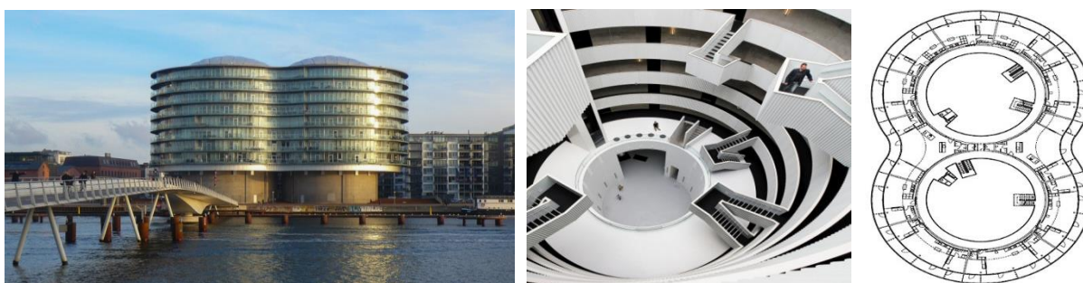
Рис. 3. Житловий комплекс «Gemini Residence» в Копенгагені, Данія; арх. «MVRDV», 2005 р.
