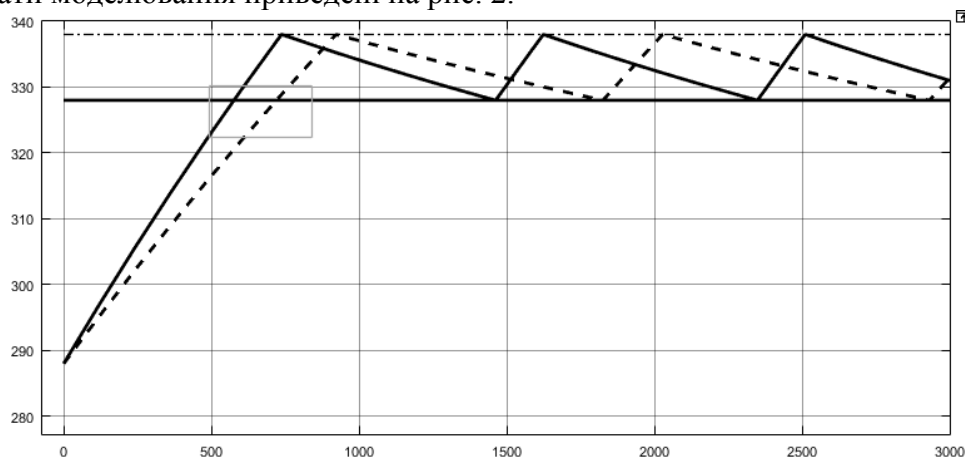
Рисунок 2 – Перебіг теплових процесів в посудомийній машині: суцільна лінія – модель без втрат тепла на посуд; штрихова лінія – модель, що враховує втрати тепла на посуд
